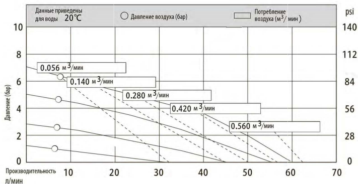
Кривые производительности насоса МК15
