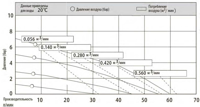
Кривые производительности насоса МК15
