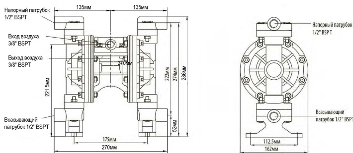
Габаритные и монтажные размеры двухлинейного насоса МК15
